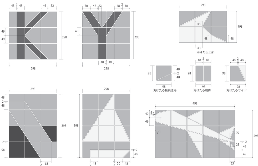
第 59 回 技能五輪全国大会 加工タイル作製説明図
